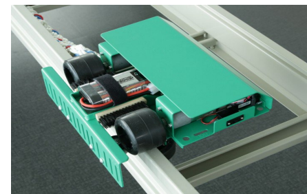
ケーブル配線用延線ロープ 布設装置「走るんですよ」
